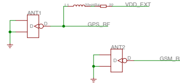
ANTENNA
